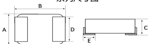
WHAA20xxxx/1770/2213 系列尺寸图
