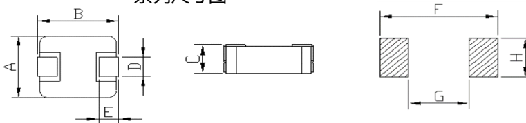
WHAA(C)0410~1265 系列尺寸图
